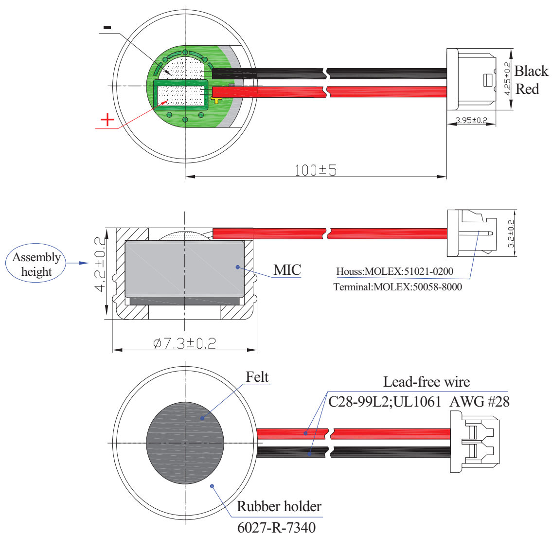
Fig. 7-1 Dimension
